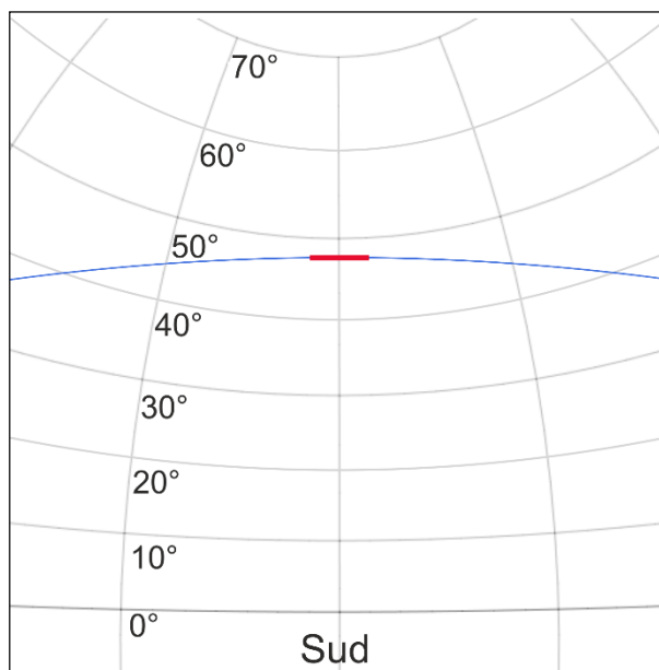
Figura 4: \varphi=43.5^\circ \text{ N} , \lambda=0^\circ , 12:00 UT asse terrestre perpendicolare all'eclittica
